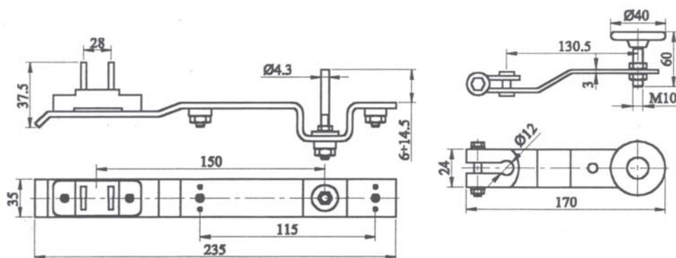
BPV-1K »D« (za desna vrata) - nacrtana BPV-1K »L« (za lijeva vrata) - zrcalna slika
