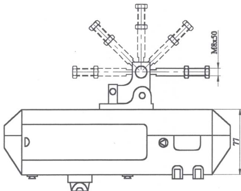
BPV-2K »D« (za desna vrata) - nacrtana
