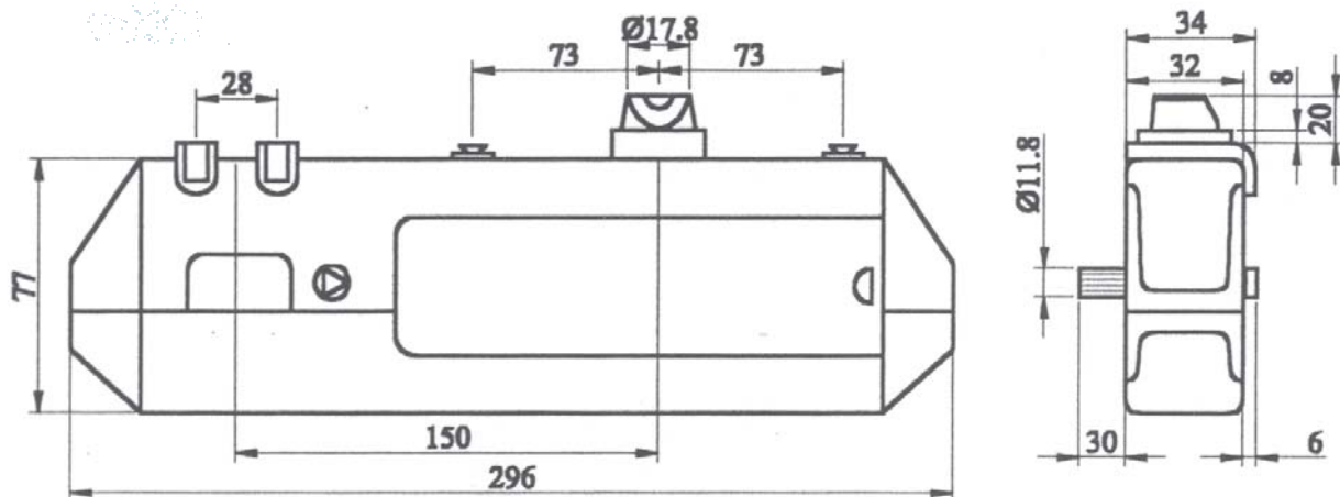
BPV-1K »D« (za desna vrata) - nacrtana BPV-1K »L« (za lijeva vrata) - zrcalna slika
