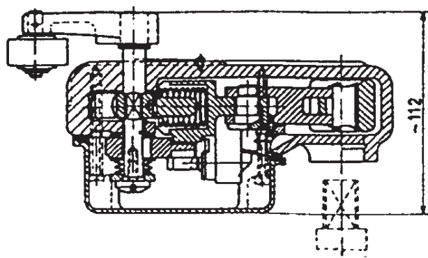
Presjek: A-B
