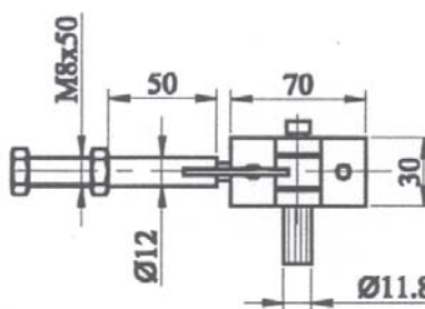
BPV-2K »D« (za desna vrata) - nacrtana
